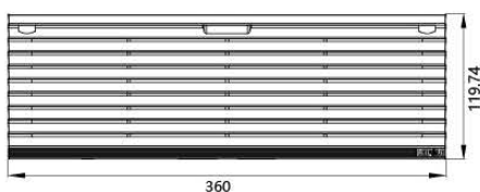
出口过滤器 FK6627.300
