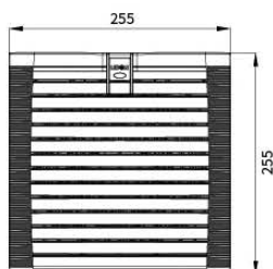
风扇及过滤器 FKL9925.230....
