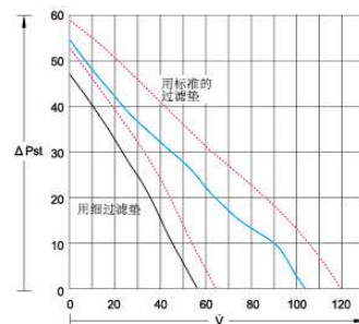
功率特性曲线 FK6627....
