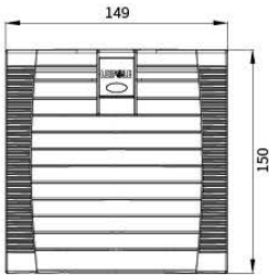
风扇及过滤器 FKL9922.230....
