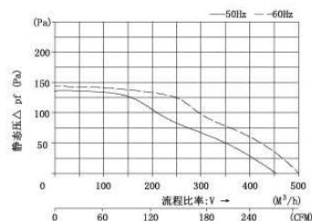
功率特性曲线 FK9926....
