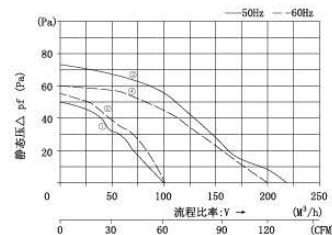
功率特性曲线 FB9804....
