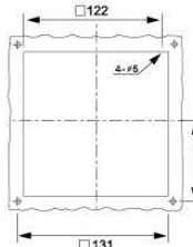
安装剖面 FB9803....
