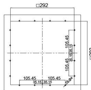
安装剖面 FKL5526-D....
