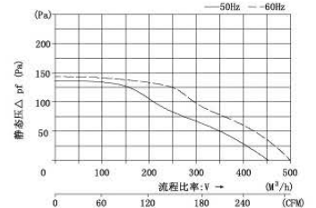
功率特性曲线 FKL6626....
