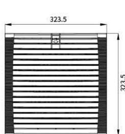
风扇及过滤器 FKL9926.230-D....
