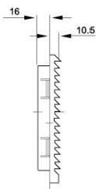
出口过滤器 FKL6622.300
