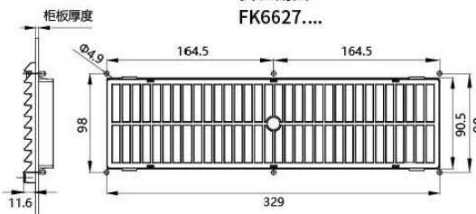
安装剖面 FK6627....
