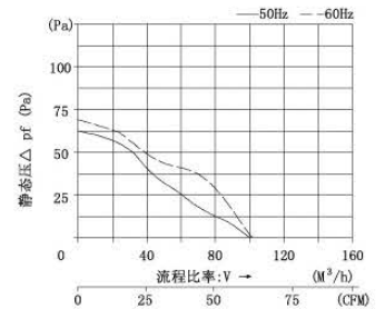
功率特性曲线 FK8923....
