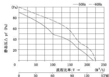
功率特性曲线 FK8925....
