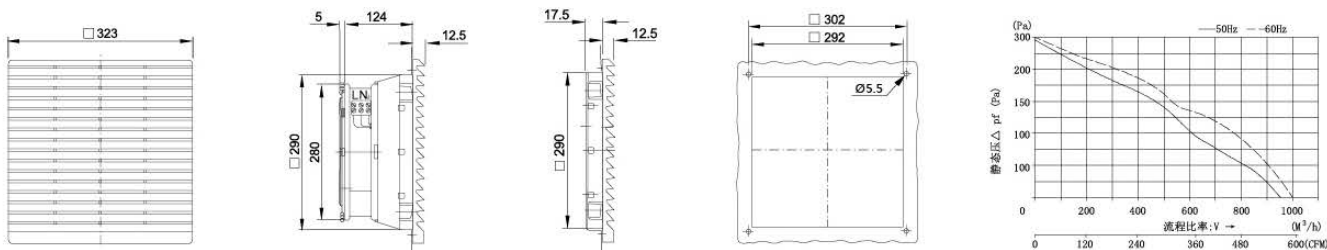
风扇及过滤器 FKL6626.230-D....
