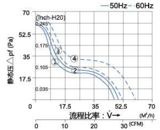
功率特性曲线 FKL6621....
