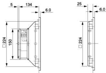
出口过滤器 FK8925.300
