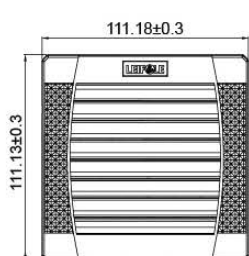
风扇及过滤器 FKL5521.024/230....
