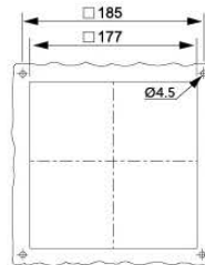
安装剖面 FKL6623....
