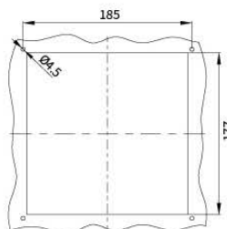
安装剖面 FKL9923-150....
