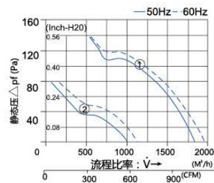
功率特性曲线 FK7726....
