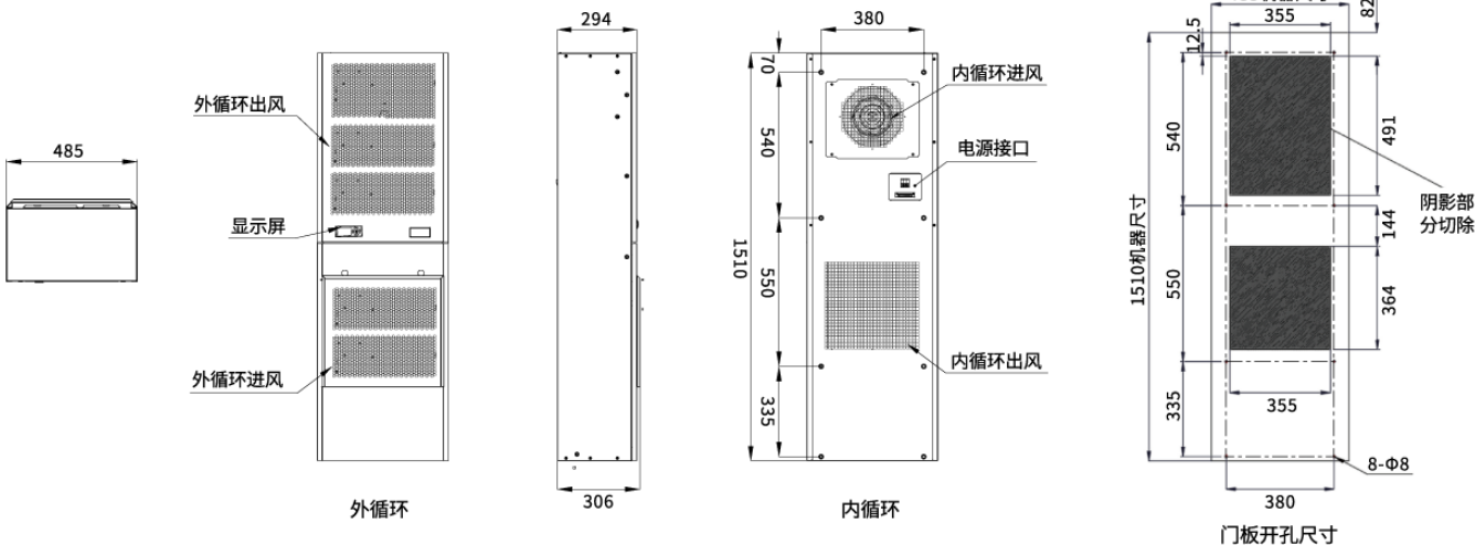
外形及门板开孔尺寸
