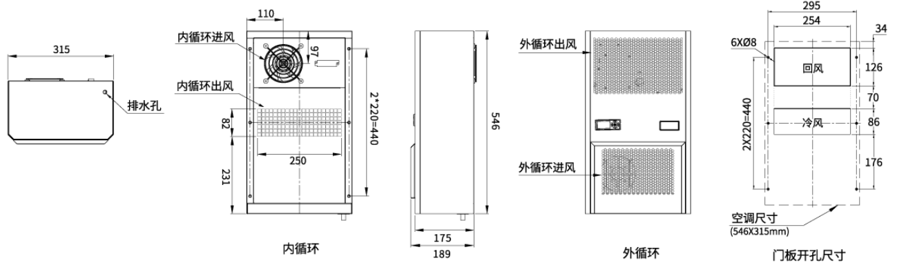
外形及门板开孔尺寸
