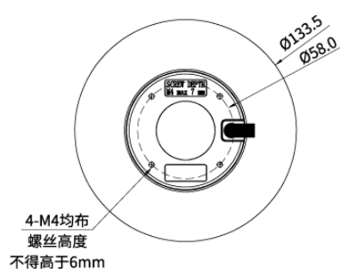
叶轮:PA6 黑色 底板:压铸铝合金
