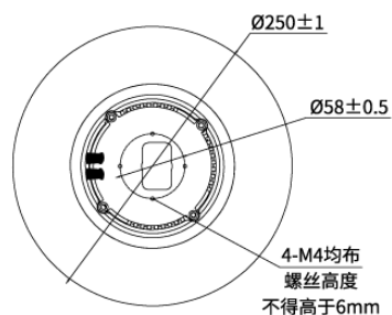
叶轮:PA6 黑色 底板:压铸铝合金
